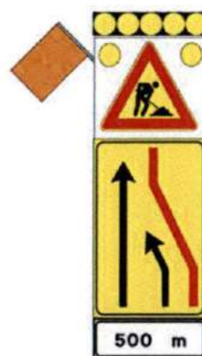
Figura 12: "segnale mobile di preavviso" fig. Il 400 Art.39 Reg. da impiegare su tratti autostradali con corsia di emergenza per la chiusura di una o più corsie di transito (la figura esemplifica la chiusura della corsia di marcia in dx). E' integrato con set di 6 lampade a led ad alta efficienza luminosa diam. 300 mm (con possibilità di lampeggio sincrono e sequenziale) e con sbandieratore elettromeccanico posto in alto sul lato esposto al traffico.
