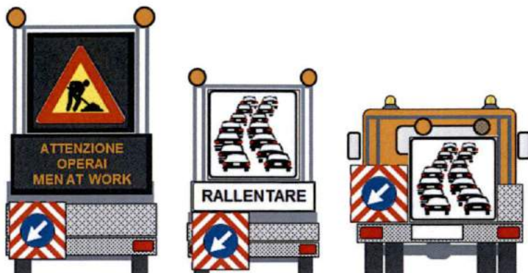
Figura 3: esempi di presegnalazione integrativa su veicolo o carrello. I pannelli "code" o "lavori in corso" devono avere dimensioni non inferiori a 120x120 cm. Il cartello Fig. II 398 Art.38 Reg. (90x90), va sempre previsto.
